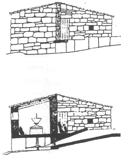
Fig. 12.- Alzado e Sección do Muiño dos Canteiros
