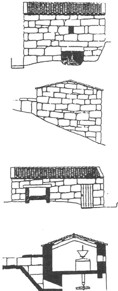
Fig. 10 .- Alzados e Sección do Muiño dos Campiños
